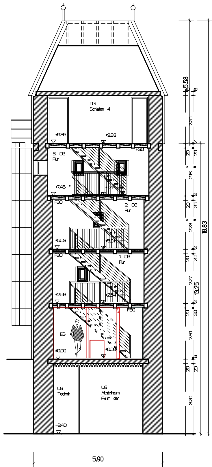
Schnitt A-A
