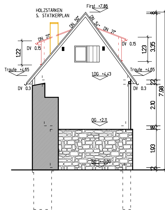
Ansicht Süd
