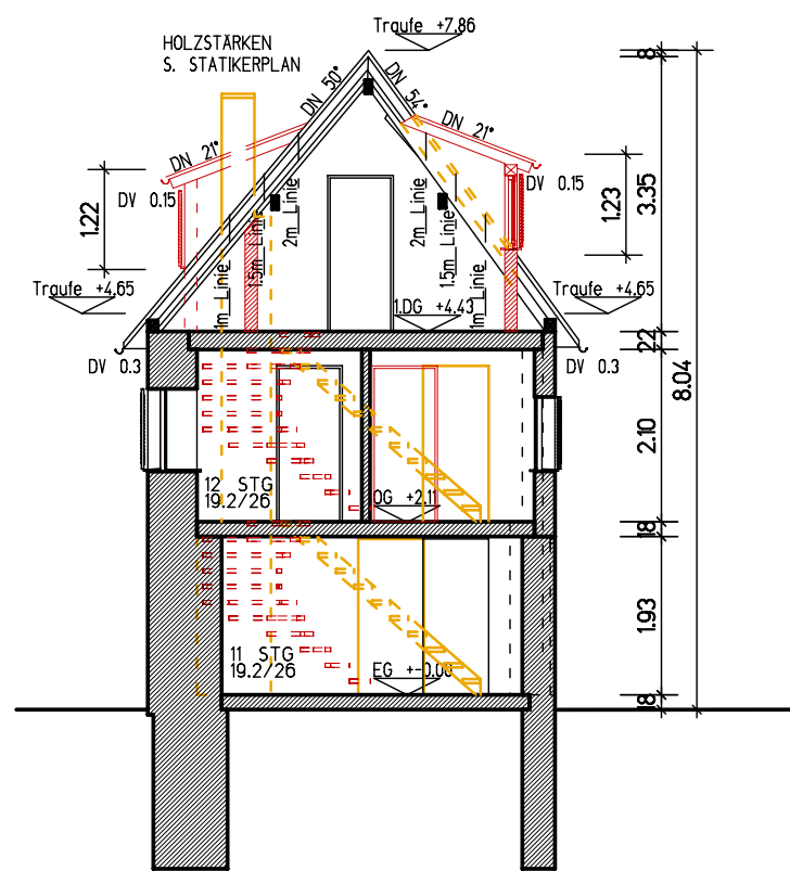
Querschnitt
