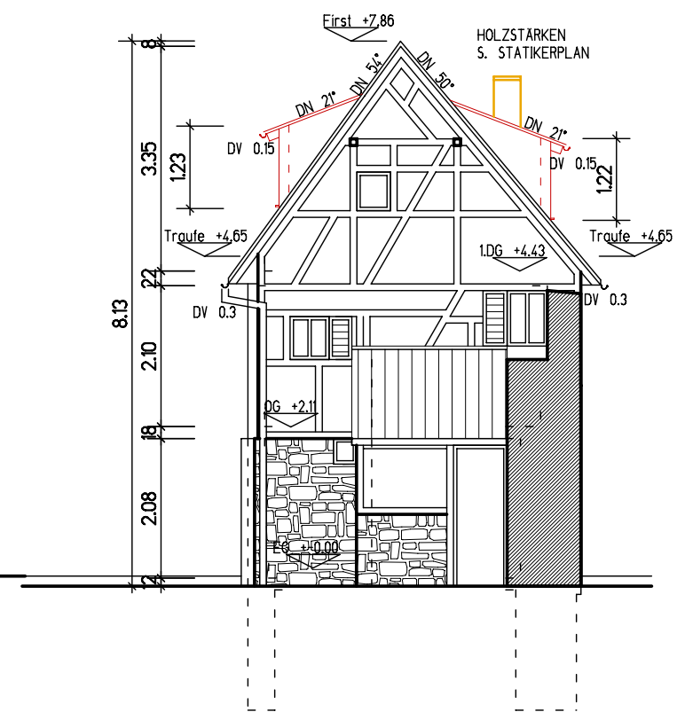
Ansicht Nord
